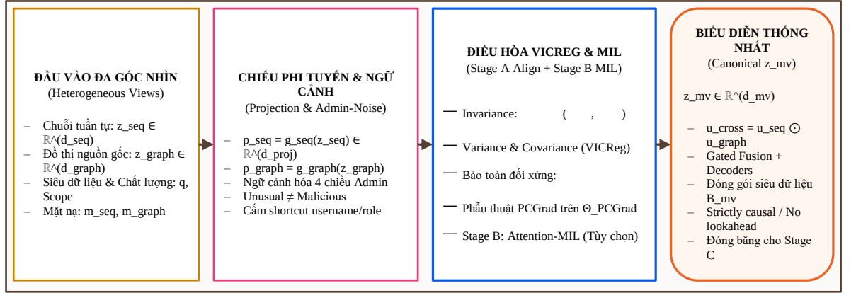
Hình 2.4: Sơ đồ kiến trúc Giống hàng đa góc nhìn, Kiểm soát sụp đổ và Tổng hợp biểu diễn thống nhất, nguồn tác giả đề xuất
