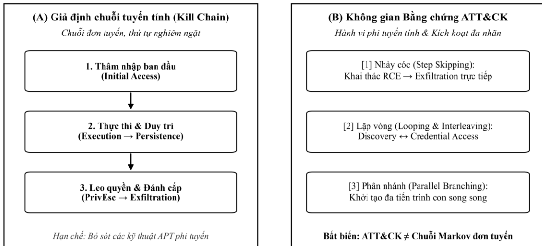
Hình 1.2: Mô hình Không gian Bằng chứng Hành vi Đa chiều MITRE ATT&CK và các đặc trưng phi tuyến tính trong tấn công APT , nguồn tác giả tổng hợp dựa trên MITRE ATT&CK [4] và Inam et al. [1]2 [6] [3]
